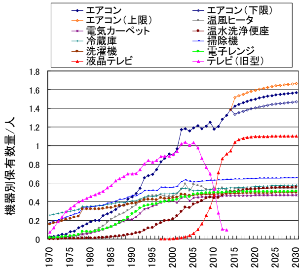
Fig.2 浦安市民が保有する家電機器数量の経年変化（エアコン上下限値は \chi^{*2} がその最小値から10%以内にある範囲を表す）
